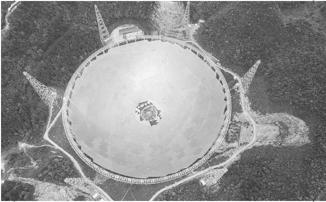
截至4月10日，正在贵州省平塘县建设的世界最大单口径射电望远镜——500米口径球面射电望远镜（FAST），已完成4185块反射面板安装，完成比例达94.04%，工程进入收尾阶段。据悉，FAST的反射面总面积约25万平方米，用于汇聚无线电波馈源接收机接收，反射面安装工程预计将于2016年5月中旬完成。 据新华社
