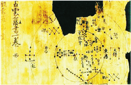
唐代天文学学生所习教材《紫微垣星图》。(见于敦煌遗书)
