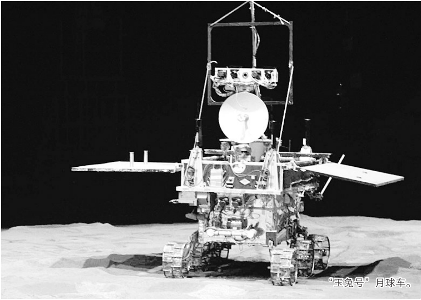
“玉兔号”是中国首辆月球车，和着陆器共同组成嫦娥三号探测器。“玉兔号”月球车设计质量140千克，能源为太阳能，能够耐受月球表面真空、强辐射、零下180摄氏度至零上150摄氏度极限温度等极端环境。月球车具备20度爬坡、20厘米越障能力，并配备有全景相机、红外成像光谱仪、测月雷达、粒子激发X射线谱仪等科学探测仪器。
